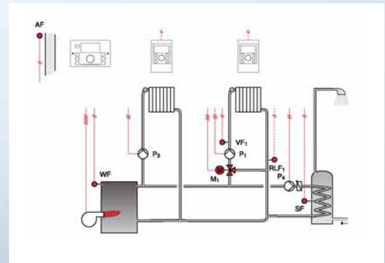
Voorbeeld: Installatie met kring radiatoren, 1 mengkring, en ketelregeling met sanitair warmwater.
