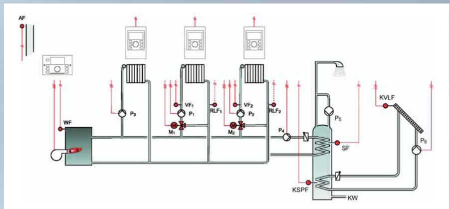
Voorbeeld: Installatie met kring radiatoren, 2 mengkringen, en ketelregeling met sanitair warmwater, inclusief zonnecollectoren.
