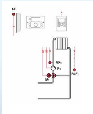
Voorbeeld: Weersafhankelijke regeling van een mengkraan
